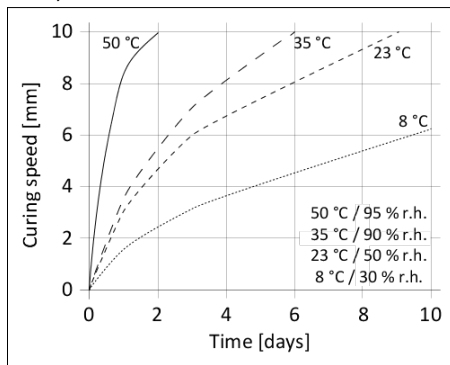
schema 1: Doorhardingssnelheid Sikasil® IG-16
