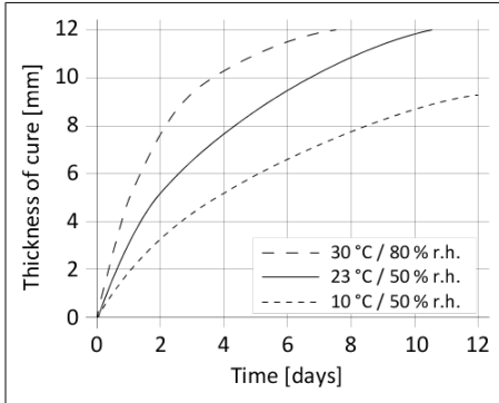
Grafiek 1: Uithardingssnelheid Sikaflex®-821 FR
